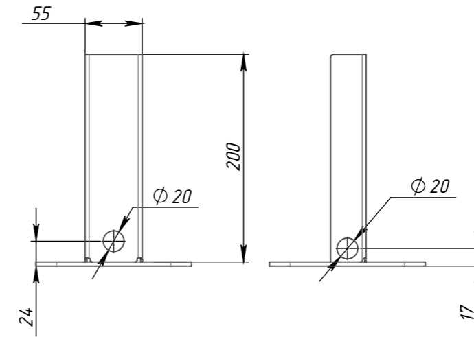
Основание с внутр. усил.
